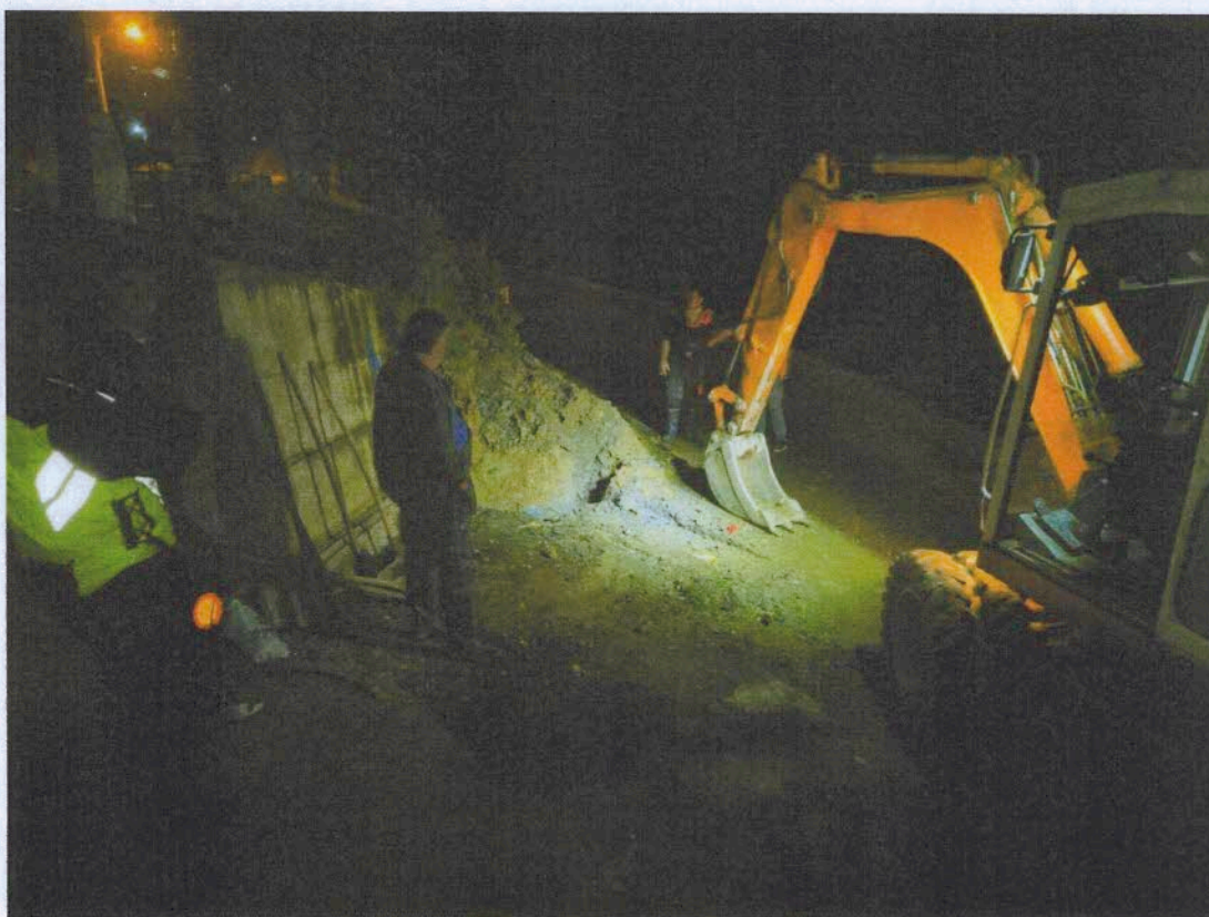
Slike: Zamjena vodovodne mreže HDPE DN 90mm u naselju Lipnica sa zamjenom priključnih cjevovoda HDPE DN 25mm
