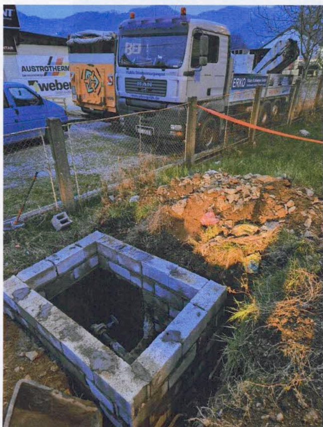
Slika: Izrada šahti na mjestima ugradnje glavnih zatvarača na sekundarnim linijama u mjestu Nedakusi i Lipnica
